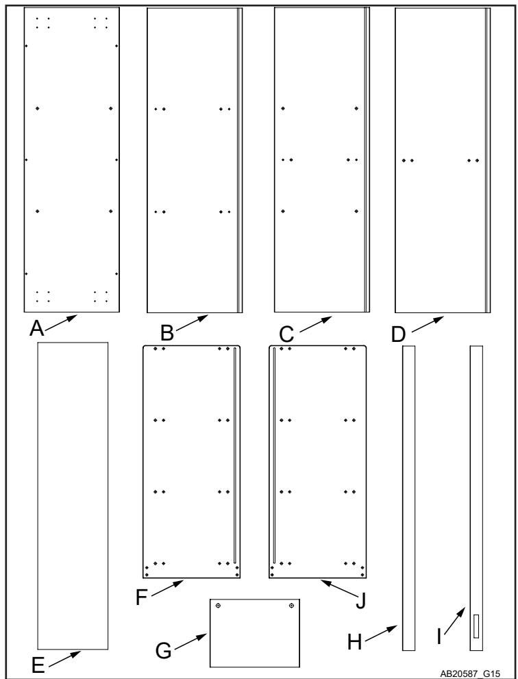
Pièces Pour Etagères de Rangement
