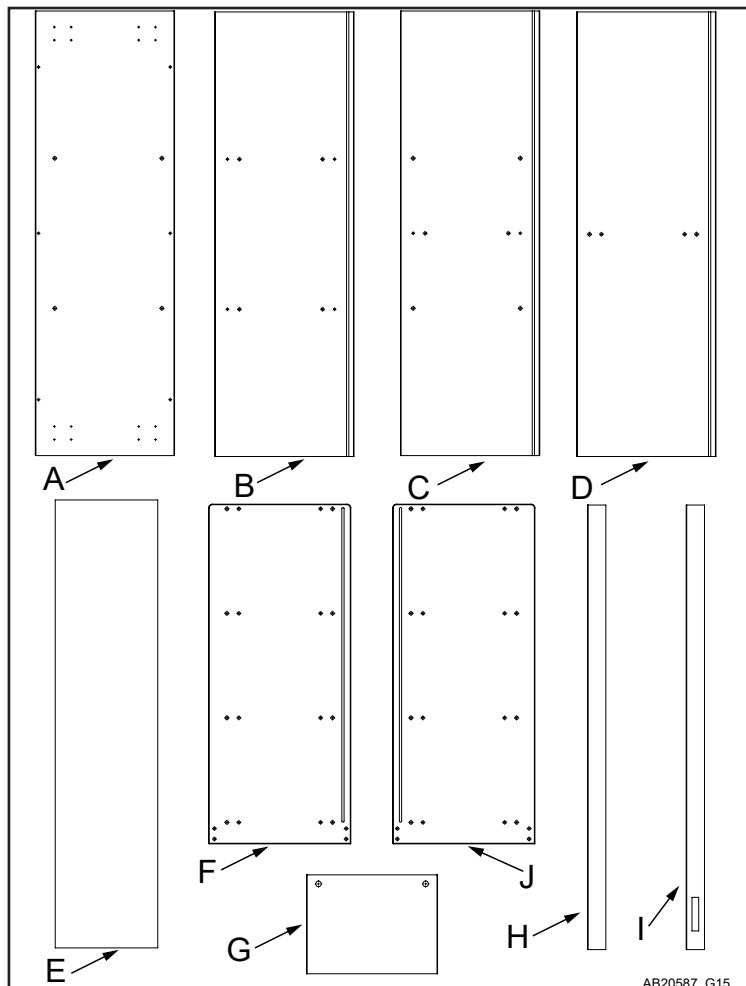
Piezas de la Unidad de Almacenamiento
